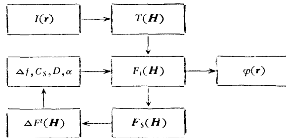
图1 计算框图
